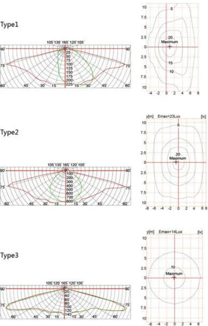
配光曲线 Polar Diagram
