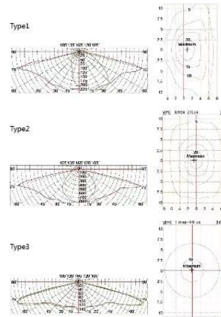
配光曲线 Polar Diagram
